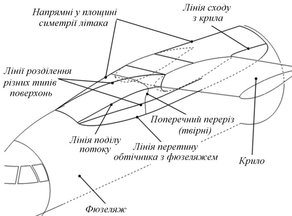
Рис. 2. Напрявні та твірні лінії обтічника
