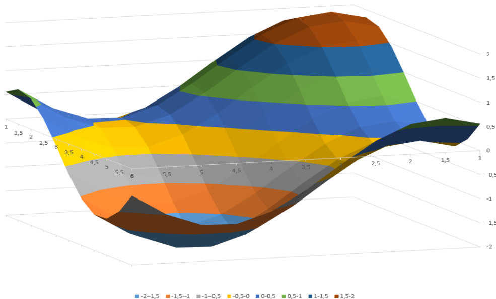
Рис. 1. Двовимірна числова послідовність z_{i,j} = \sin i + \sin j
