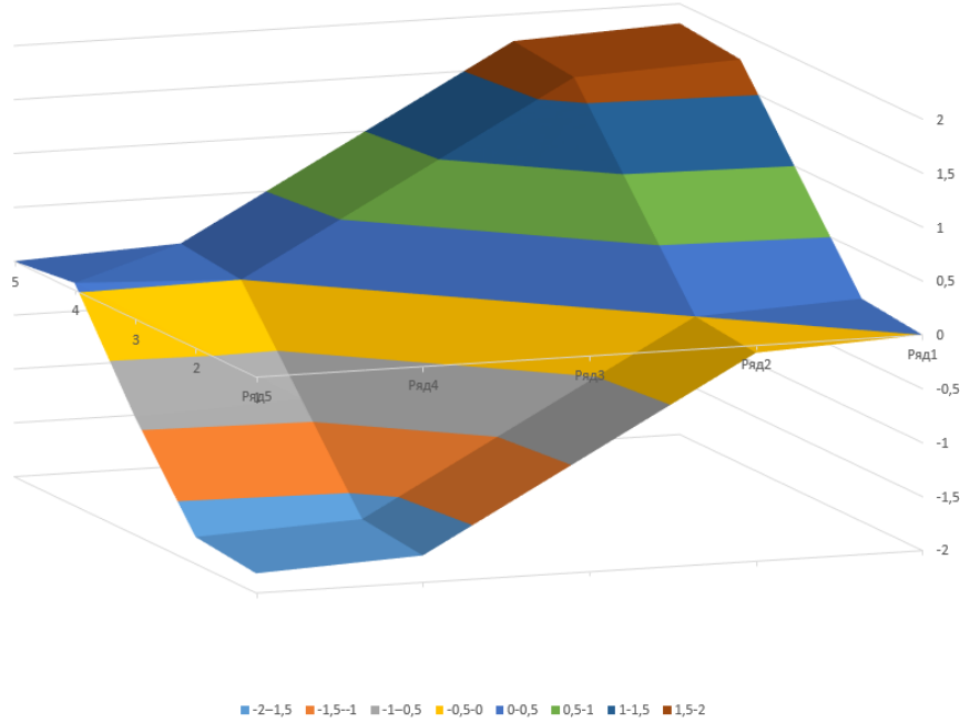
Рис. 3. Дискретний каркас поверхні z_{i,j} = \sin i + \sin j
