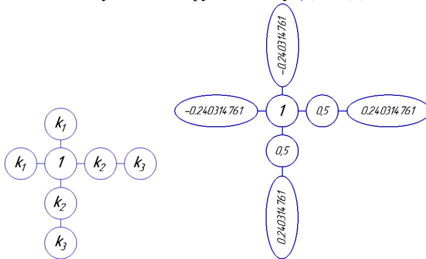
Рис. 2. Обчислювальний шаблон для дискретної інтерполяції числовою послідовністю двох змінних z_{i,j} = \sin i + \sin j
