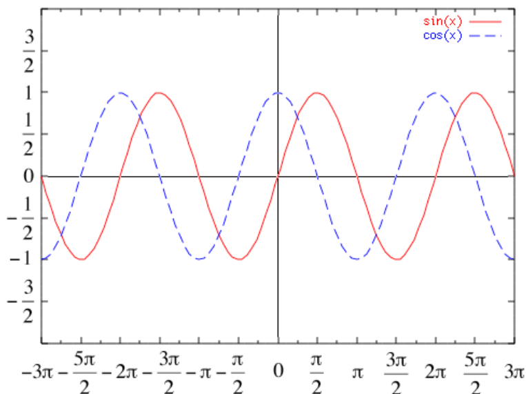
Рис. 1. Графіки синусоїд.
