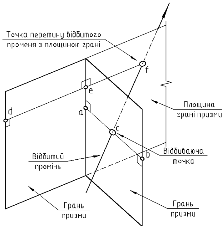
Рис. 3. До визначення грані, яка буде відбивати промінь
