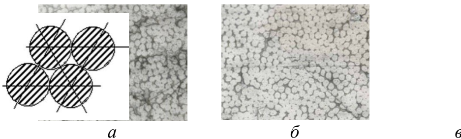
Рис. 6. Типова фотографія мікрошліфу поперечного перерізу затверділого орієнтованого епоксидного органопластика: а – до УЗ-обробки; б – після УЗ-обробки; в – гексагональна (теоретична)
