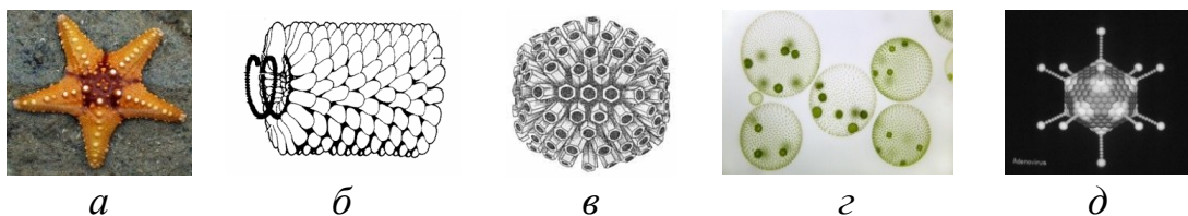
Рис. 2. Приклади симетрій: a – аксіальна; б – спіральна (вірус табачної мозаїки); в – кубічна (вірус герпеса); г – сферична (вольвокс); д – ікосаедрична (капсид аденовіруса ) [5]
