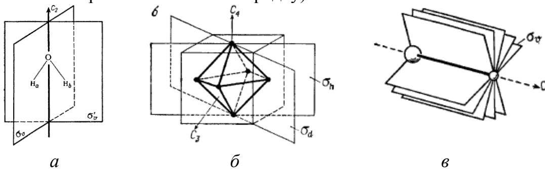
Рис. 3. Елементи симетрії: a – молекули води; б – кубічної; в – неперервної; c_n – вісь симетрії n -го порядку, \sigma_v і \sigma_h – відповідно, вертикальна і горизонтальна площини симетрії [6]
