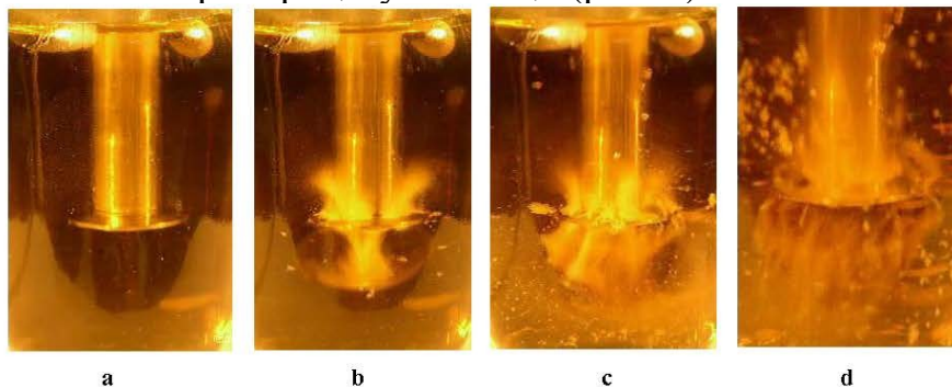
Рис. 5. Зародження і розвиток УЗ-кавітації в рідкому епоксидному олігомері марки ЕД-20 під час обробки концентратором
