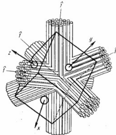
Рис.4. Чотирьохспрямована схема армування та розташування системи координат; x, y, z – головні осі пружної симетрії; \hat{f} – напрямок армування [7]
