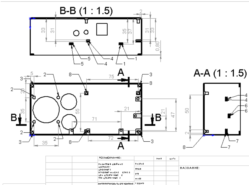
Рис. 4. Приклад збірного креслення корпусу блока управління
