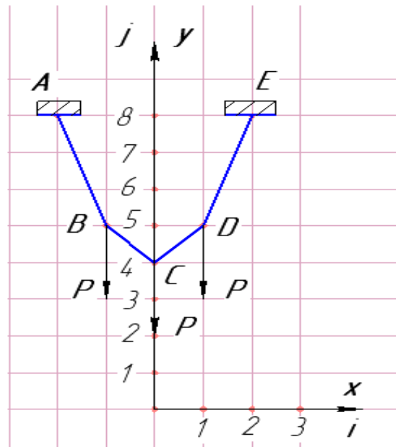
Рис. 1. Дискретно представлена крива (ДПК) y = x^2 + 4 .
